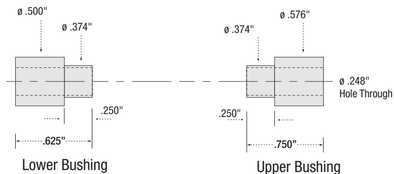
DIAGRAM D • PKSPCL2BU
